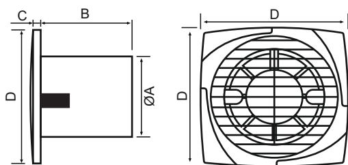
Motor sa termičkom zaštitom Motor with thermal protection
