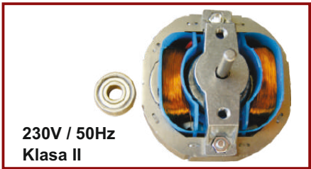
230V / 50Hz Klasa II Motor sa termičkom zaštitom (sa ležajem) Motor with thermal protection (with bearing)
