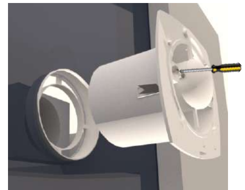
Brzim zatezanjem žabica u odgovarajući otvor za modele A100MX-S Fast installation by tightening hooks into matching hole
